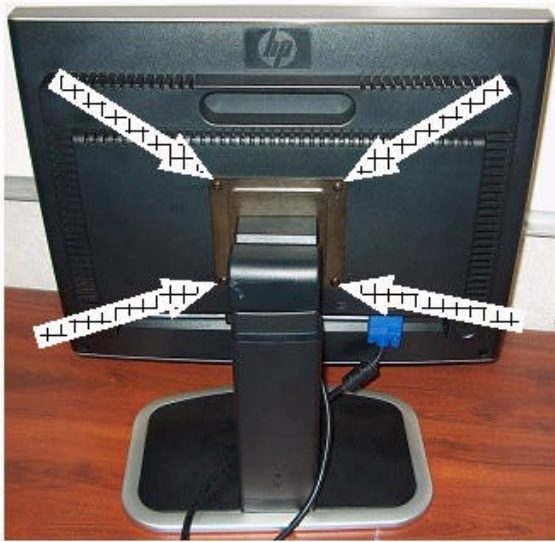
Figura 1a: Staffa di montaggio del supporto del monitor L2035
